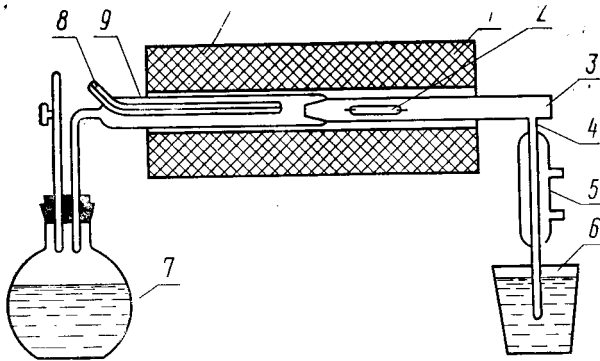
Схема пирогидролитической установки
